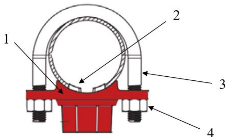
Ryc. 5. Konstrukcja króćca rurowego nakładkowego typu 041.
