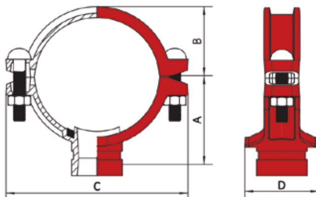
Ryc. 4. Konstrukcja króćca rurowego nakładkowego typu XGQT04G. Źródło: Materiały producenta.
