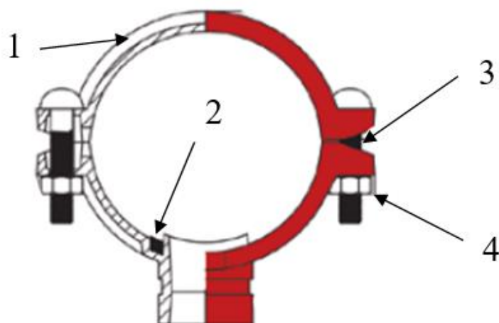
Ryc. 6. Konstrukcja króćca rurowego nakładkowego (na przykładzie króćca rurowego typu XGQT04G).
