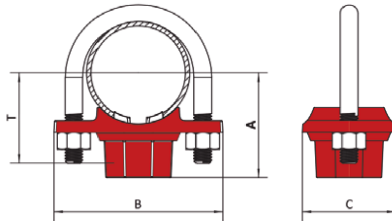
Ryc. 1. Wymiary króćca rurowego nakładkowego typu 041. Źródło: Materiały producenta.
