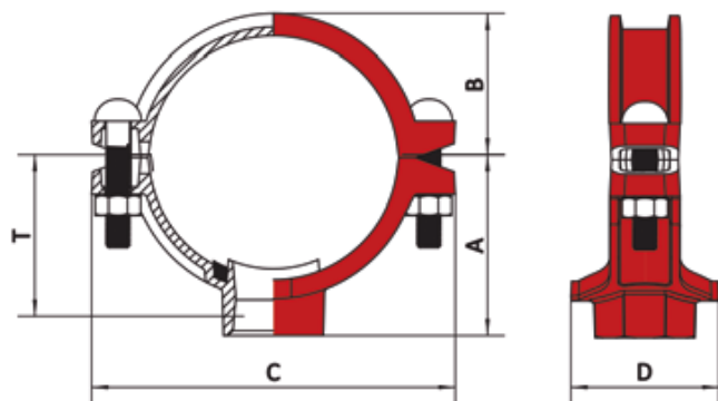
Ryc. 3. Konstrukcja króćca rurowego nakładkowego typu XGQT04.
