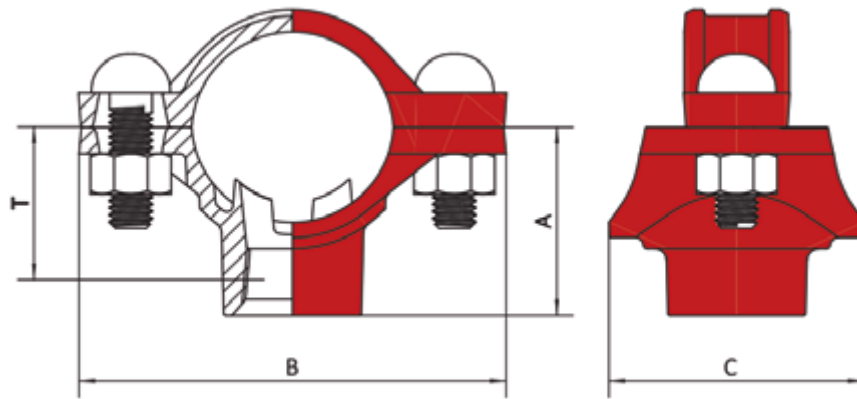
Ryc. 2. Wymiary króćca rurowego nakładkowego typu L922. Źródło: Materiały producenta.
